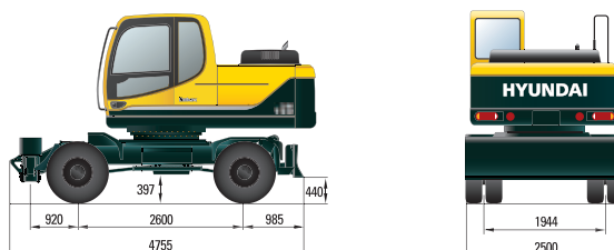
HW140 AVEC LAME DE BOUTEUR ARRIÈRE ET STABILISATEURS AVANT
