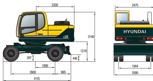
HW140 AVEC LAME DE BOUTEUR ARRIÈRE
