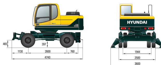
HW140 AVEC STABILISATEURS ARRIÈRE ET LAME DE BOUTEUR AVANT
